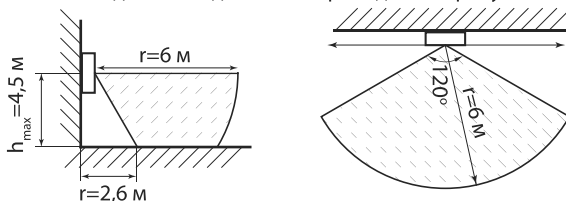
Рисунок 1. Зона обнаружения датчиком движения
